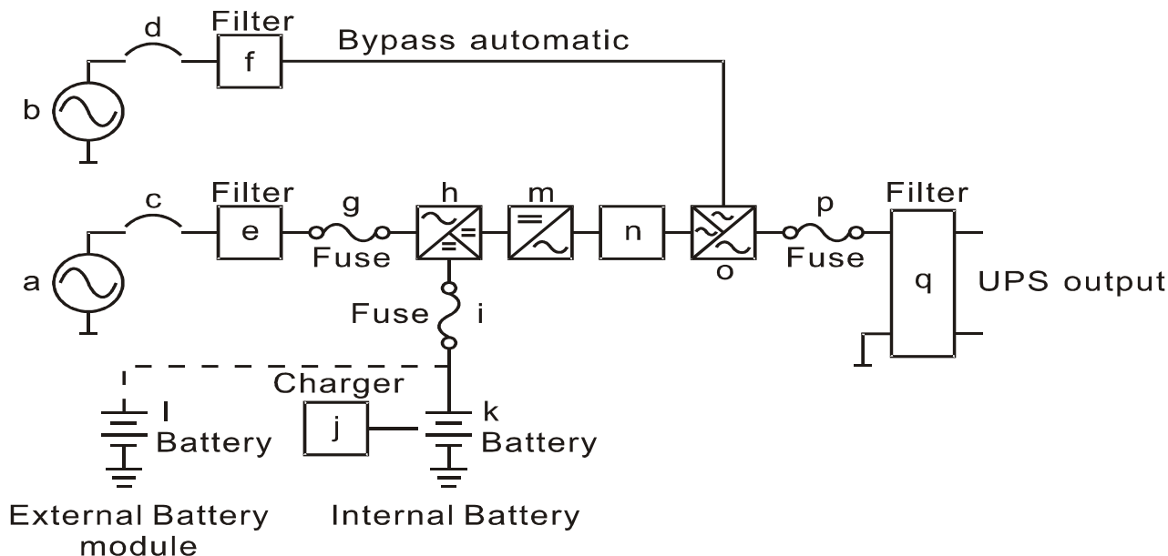
Рис.3.1-1 Блок-схема ИБП Monolith 20000RT-31
