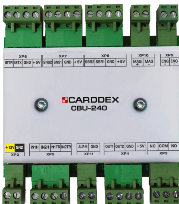
Рисунок 6.3.1 Контроллер управления турникетом «CBU-240»
