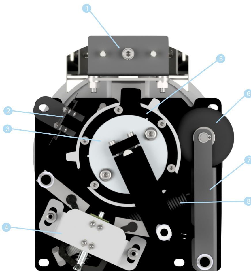
Рисунок 6.2.1 Внутренний механизм ТМ-2 турникета «STL-03»
