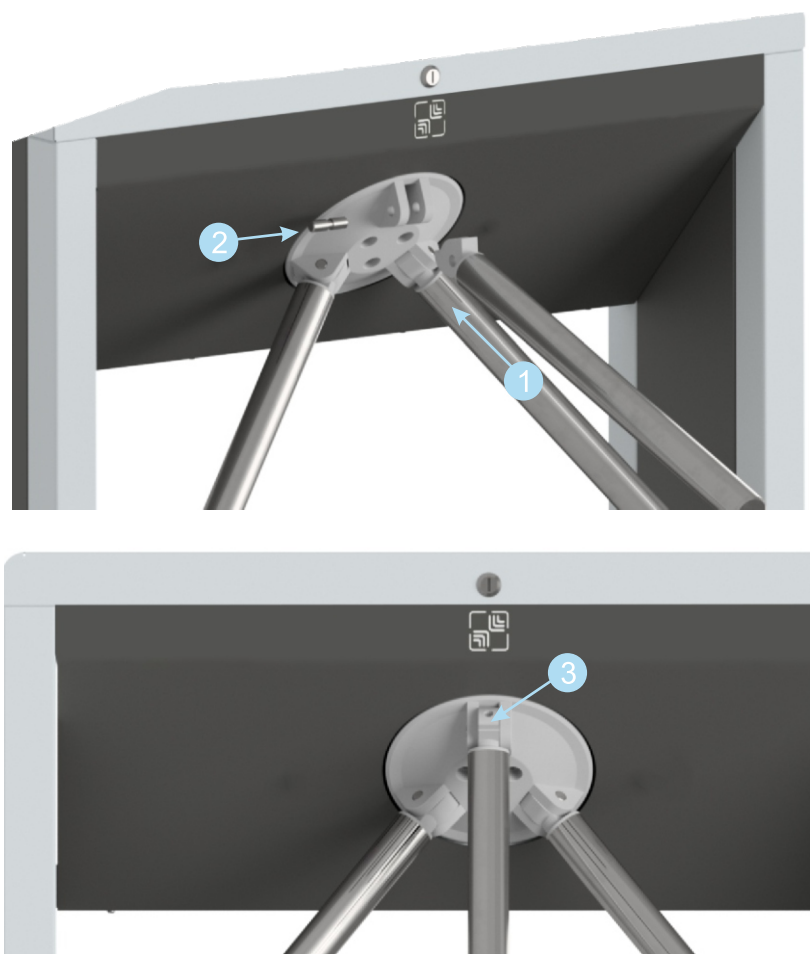
Рисунок 7.5.1 Установка преграждающих планок
