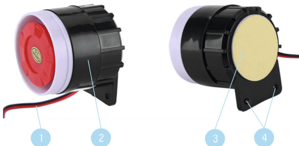
Рисунок 6.7.2 Излучатель звука (сирена)
