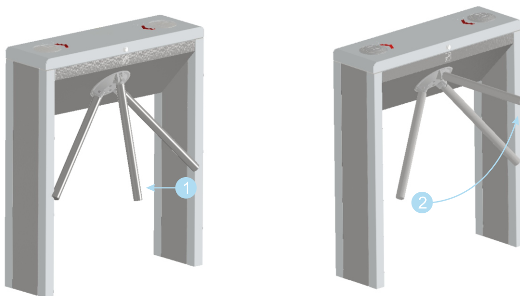
Рисунок 6.5.3 Установка планок в положение блокировки прохода
