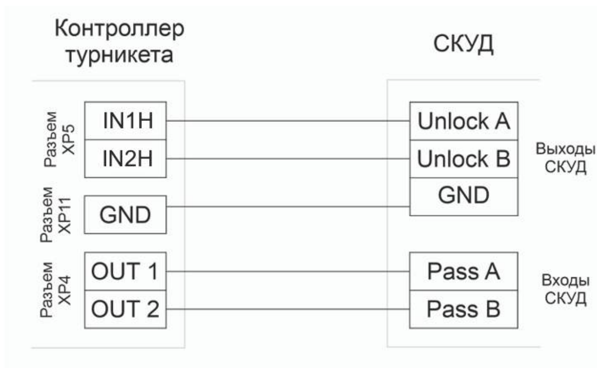
Рисунок 8.2.1 - Подключение турникета к стороннему СКУД
