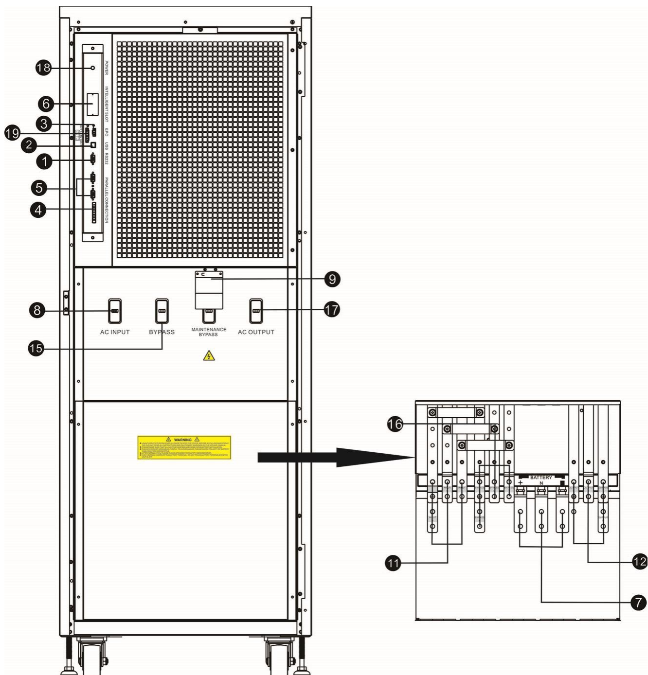
Рисунок 3. Передняя панель(дверь открыта) и клеммы подключения XF100/120
