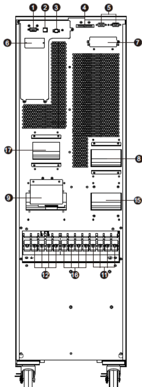
Рисунок 1. Задняя панель и клеммы подключения XF40(wb)
