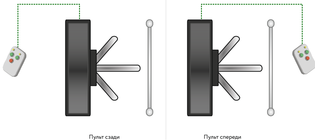
Рисунок 4.2 – Расположение пульта относительно турникета 3V
