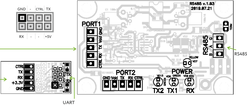
Рисунок 5.2 - Плата RS485
