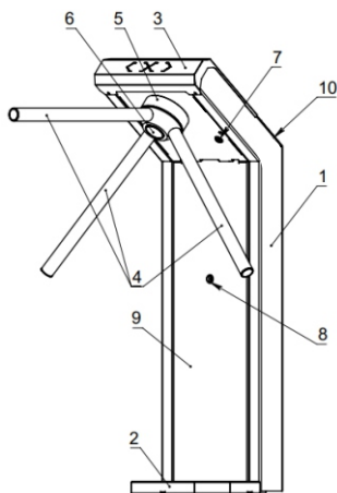
Рисунок 1.6 – Турникет-трипод (напольный) «3V Model V / V(i)*»
