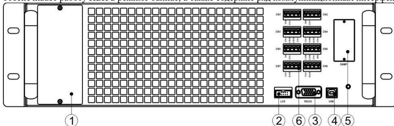
Рисунок 11. Модуль байпаса.
