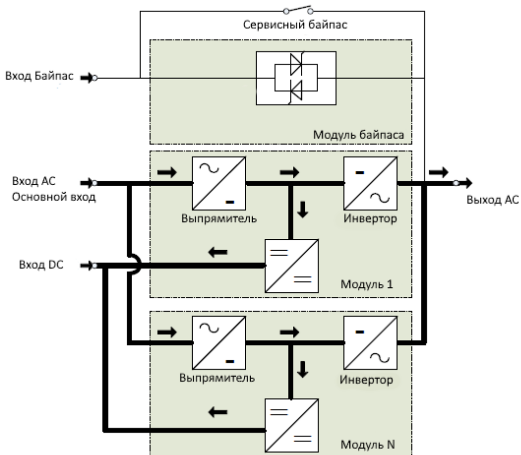
Рисунок 13. Нормальный режим
