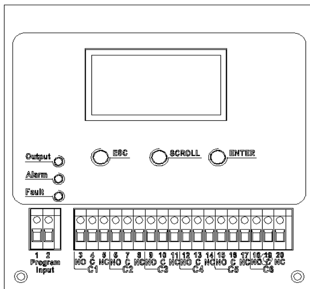
Рис.5 Лицевая панель.
