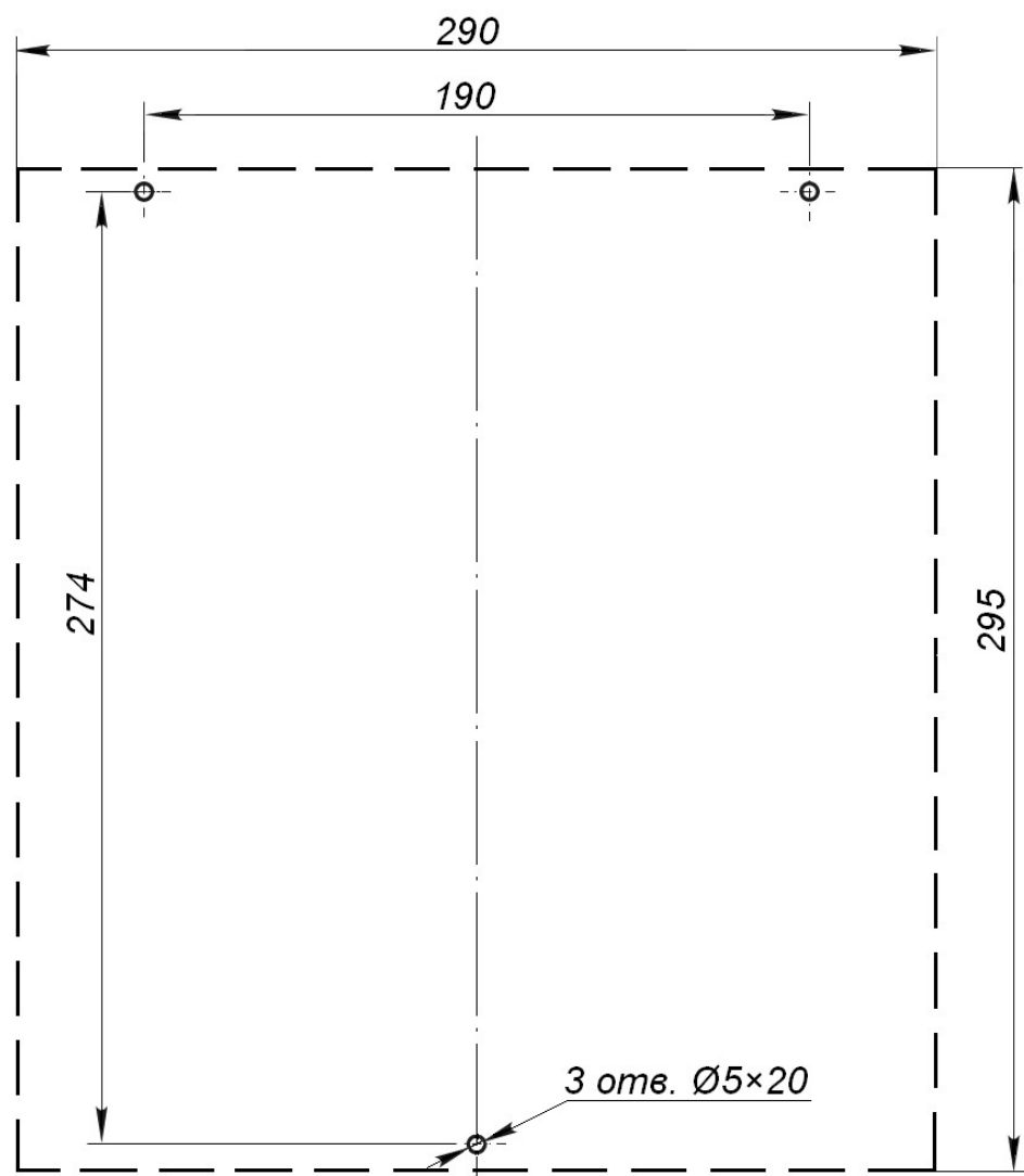
Рисунок 9. Разметка отверстий для крепления БУ на стене
