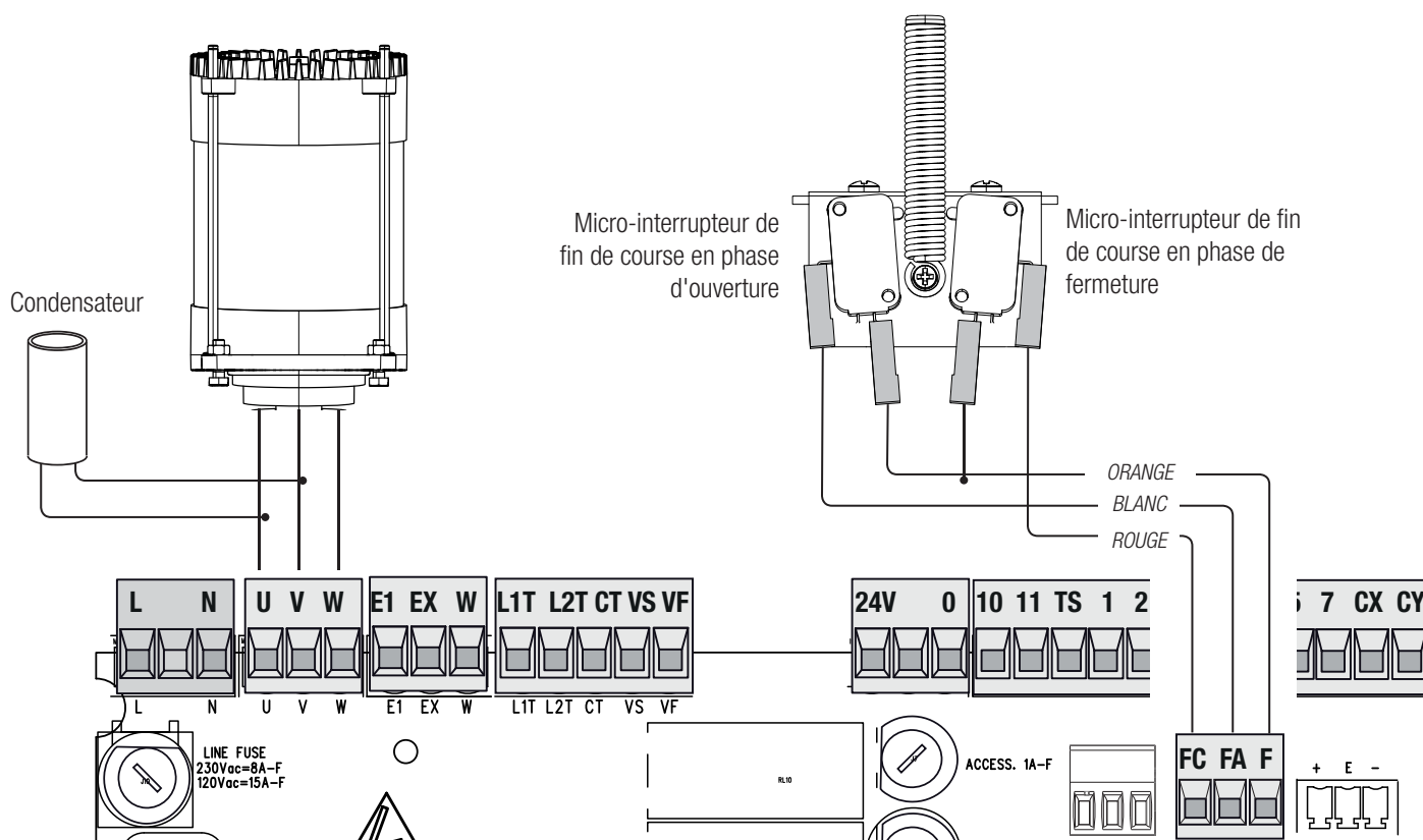
Motoréducteur 120/230 VAC
